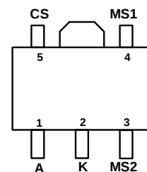
SOT-89- 5L
