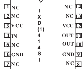
14 PIN SOIC
