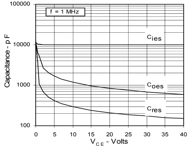
Fig. 12. Capacitance
