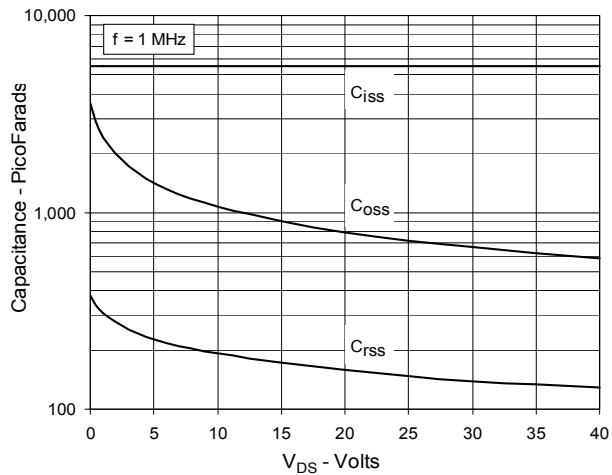
Fig. 11. Capacitance
