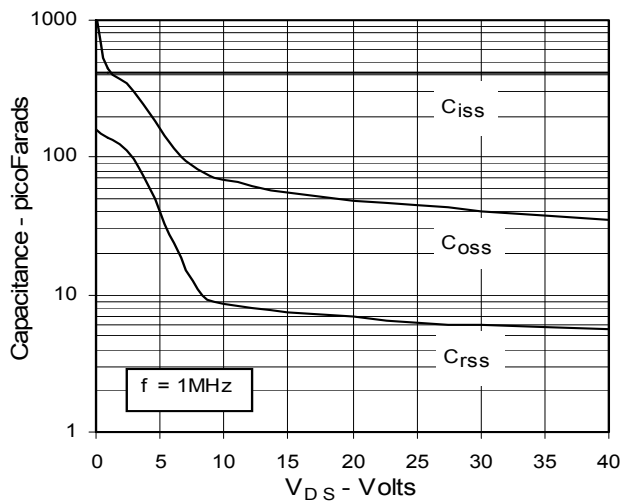
Fig. 11. Capacitance
