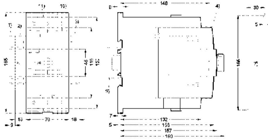
Circuit-breaker J7MN-100
