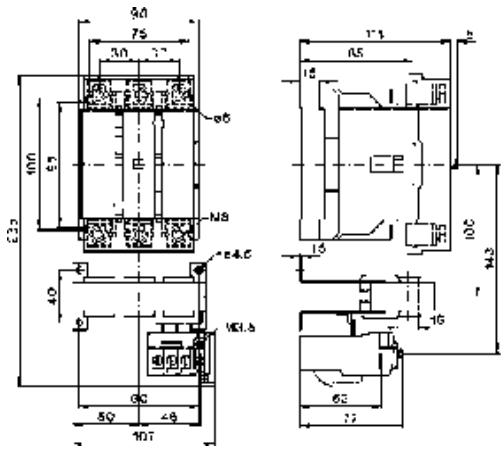
J7KN-200 + J7TKN-210
