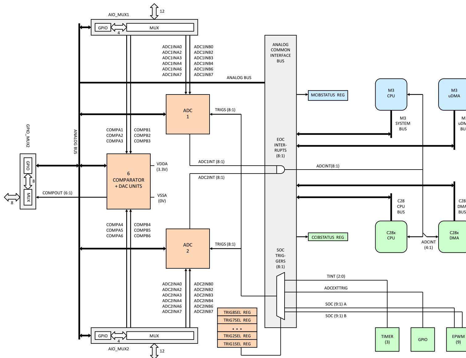
图 6-3. Analog Subsystem
