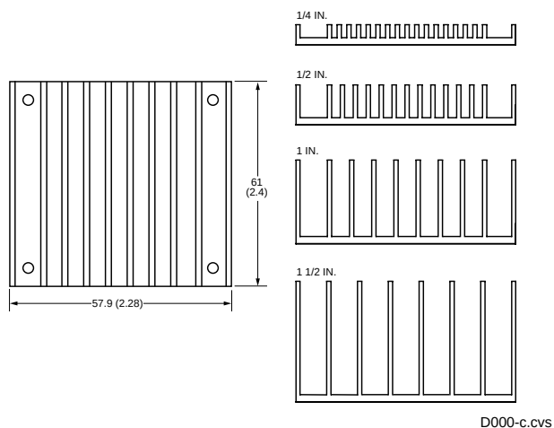
Figure 38. Longitudinal Heat Sink
