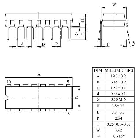
DIP-16
