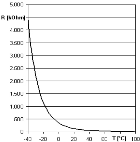
Typical Thermistor Graph 5) page 20 , 6) page 20 Typische Thermistor Kennlinie 5) Seite 20 , 6) Seite 20
