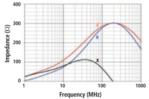
29F0430-4SR-10
