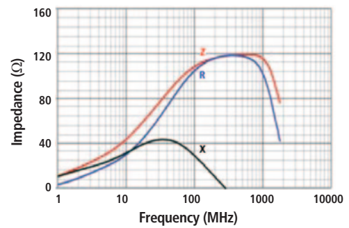
29F0418-1SR-10, 29F0818-1SR-10
