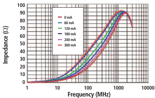
LI0402C470R-10
