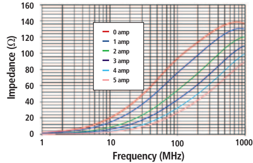
HI1812V101R-10
