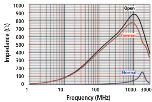
CM0805A371R-10
