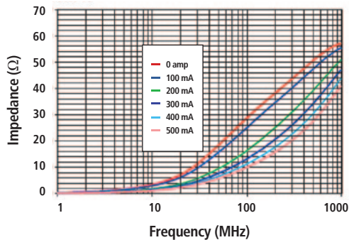
LI0402E300R-10
