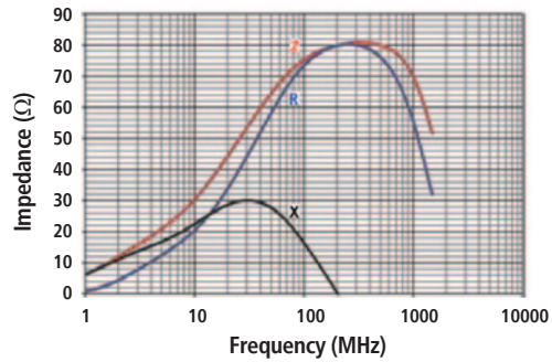
29F0418-0SR-10, 29F0818-0SR-10
