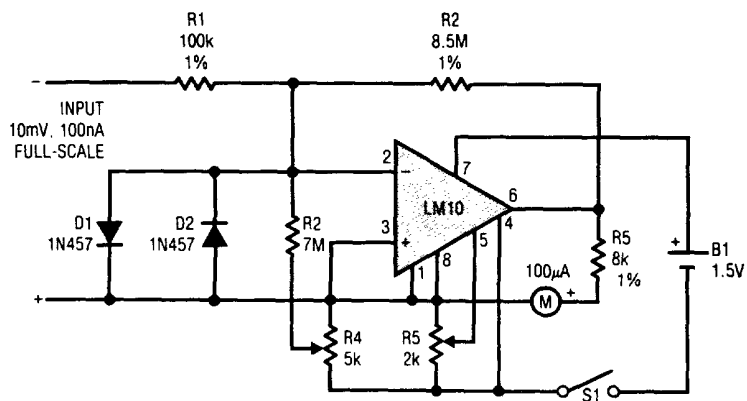
Meter Amplifier
