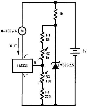
0°C–100°C Thermomemter
