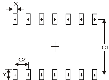
SO-14
