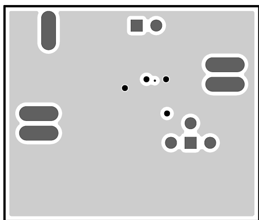
Layer 2 (GND)
