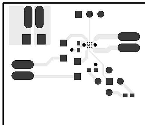
Top Layer
