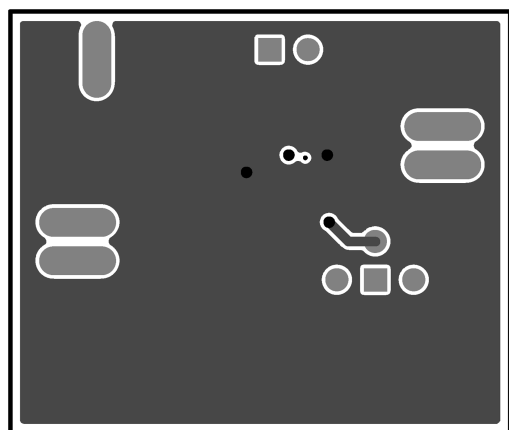
Bottom Layer
