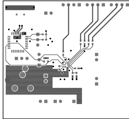
Bottom Layer
