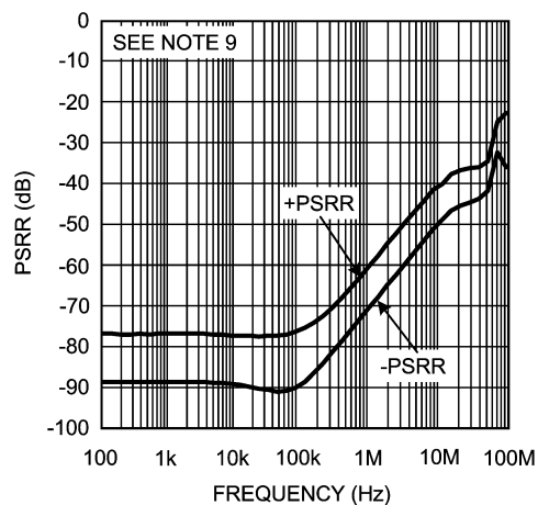
PSRR
