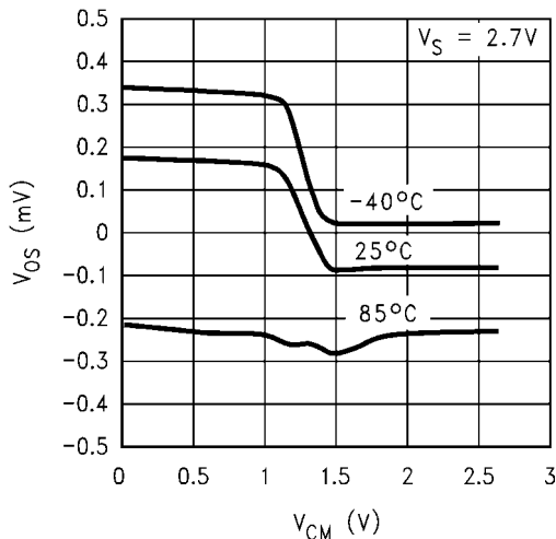
V_{OS} vs. V_{CM}
