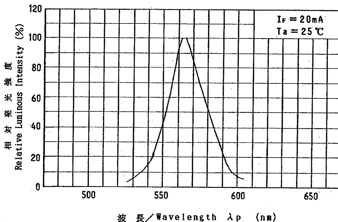
相对発光強度 — 波長特性 Relative Luminous Intensity Wavelength Characteristics
