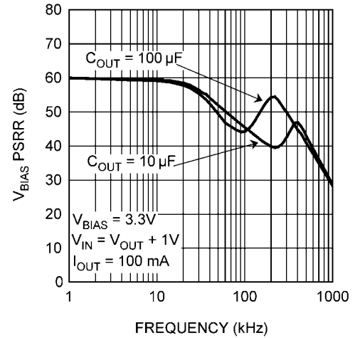
V_{BIAS} PSRR
