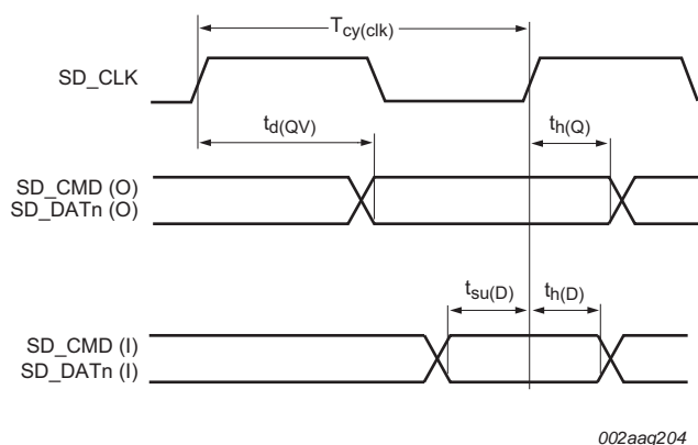
Fig 30. SD/MMC timing
