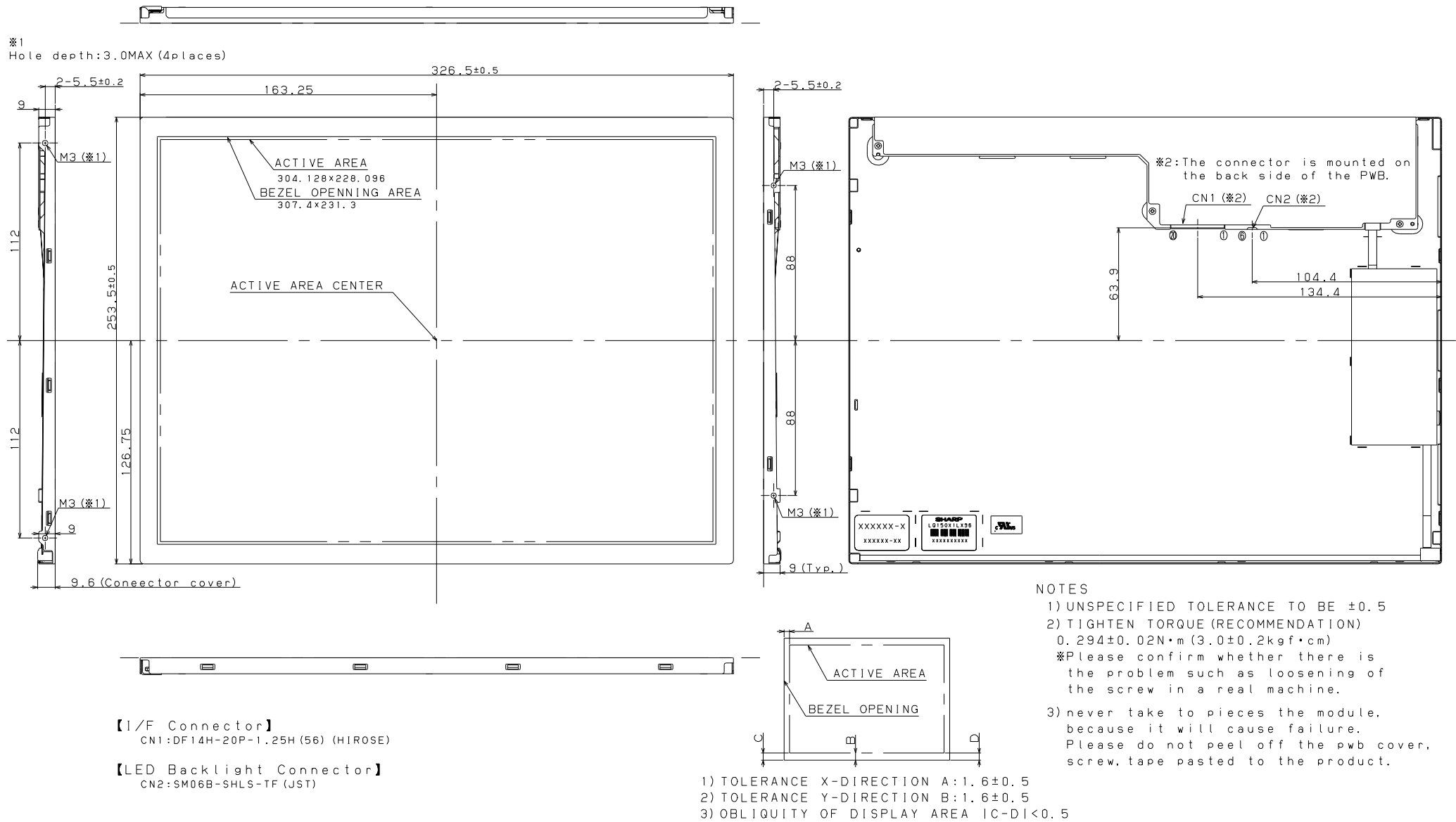
图1. LQ150X1LX96外形寸法图 Fig.1. Outline Dimensions
