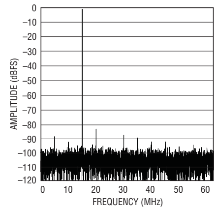
LTC2268-12: 8k Point FFT, f_{IN} = 140\text{MHz} , -1\text{dBFS} , 125\text{Msps}
