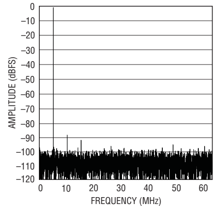
LTC2268-12: 8k Point FFT, f_{IN} = 5\text{MHz} , -1\text{dBFS} , 125\text{Msps}
