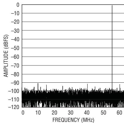
LTC2268-12: 8k Point FFT, f_{IN} = 70\text{MHz} , -1\text{dBFS} , 125\text{Msps}
