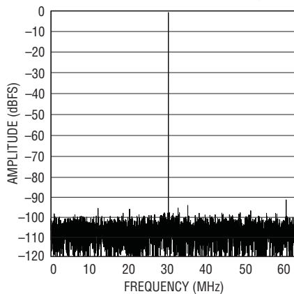
LTC2268-12: 8k Point FFT, f_{IN} = 30\text{MHz} , -1\text{dBFS} , 125\text{Msps}
