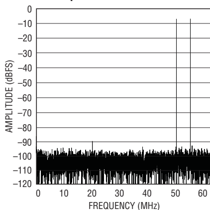
LTC2268-12: 8k Point 2-Tone FFT, f_{IN} = 70\text{MHz} , 75\text{MHz} , -1\text{dBFS} , 125\text{Msps}
