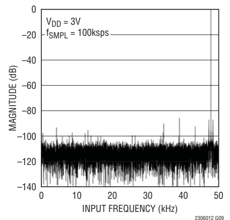
48kHz Sine Wave 8192 FFT Plot
