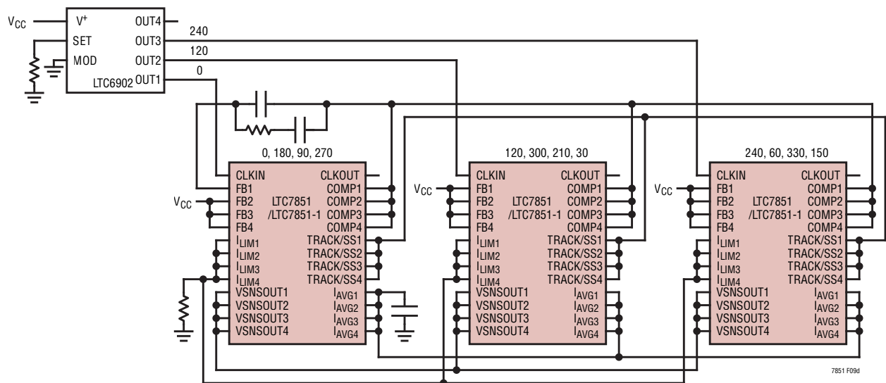
(d) 12-Phase
