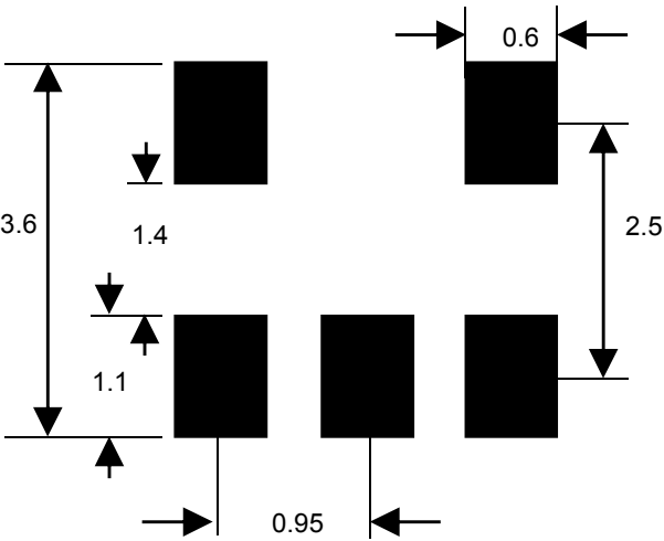
Package : SOT23-5L
