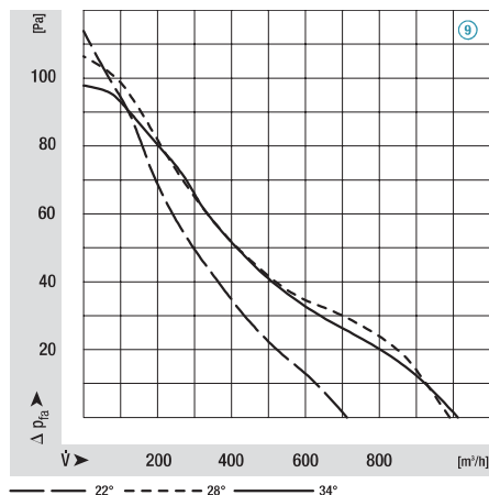
M4Q045-DA01-**, Ø 254, 50 Hz
