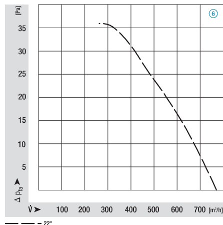
M4Q045-CA03-**, Ø 254, 60 Hz
