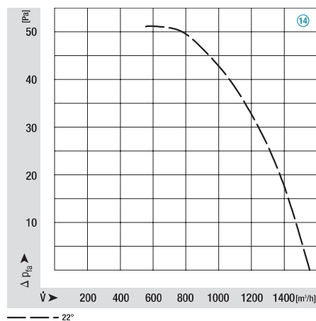
M4Q045-EA01-**-**, Ø 300, 60 Hz
