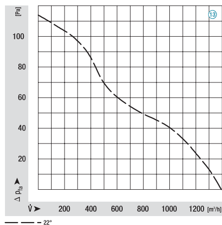
M4Q045-EA01-**-**, Ø 300, 50 Hz
