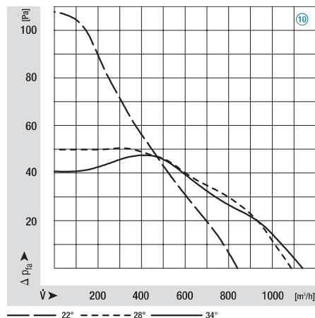
M4Q045-DA01-**, Ø 254, 60 Hz
