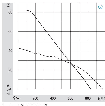
M4Q045-CF01-**, Ø 254, 60 Hz
