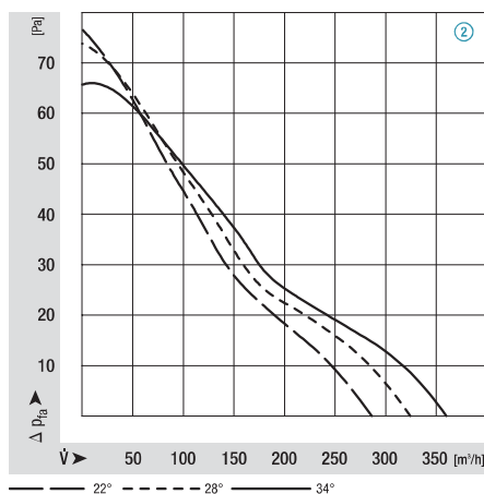
M4Q045-BD01-**, Ø 172, 60 Hz
