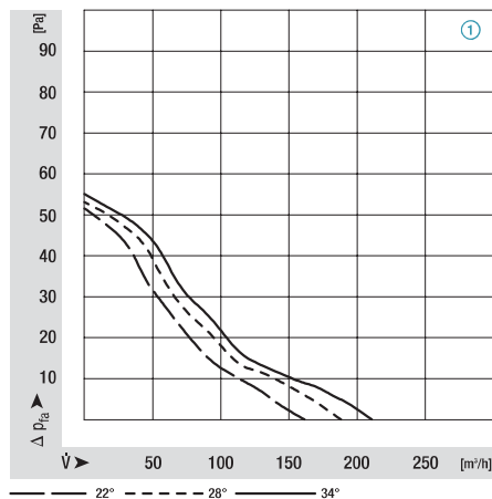
M4Q045-BD01-**, Ø 154, 50 Hz
