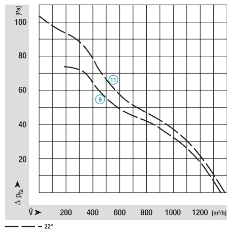
⑨ M4Q045-DA01-**-** / ⑪-DA05-**-**, Ø 300, 50 Hz
