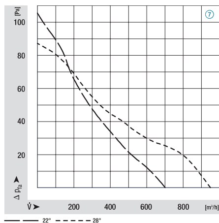
M4Q045-CF01-**, Ø 254, 50 Hz
