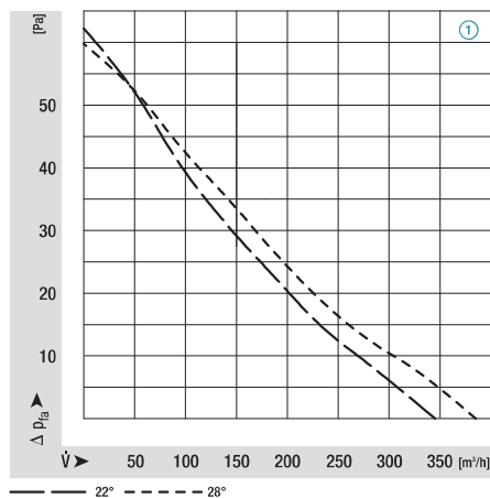
M4Q045-BD01-**, Ø 200, 50 Hz
