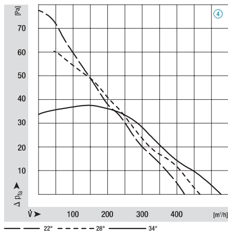
M4Q045-CA01-**, Ø 200, 60 Hz
