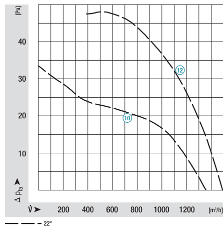
⑩ M4Q045-DA01-**-** / ⑫-DA05-**-**, Ø 300, 60 Hz
