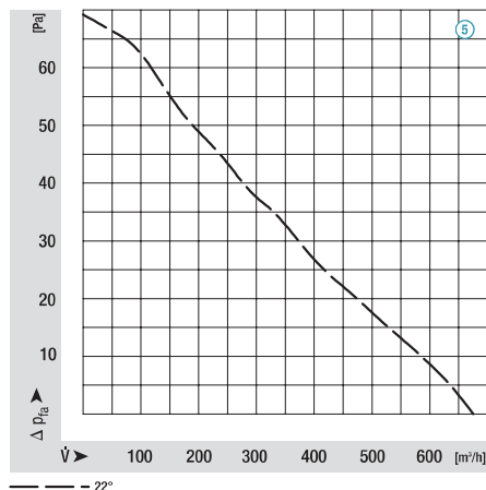
M4Q045-CA03-**, Ø 254, 50 Hz
