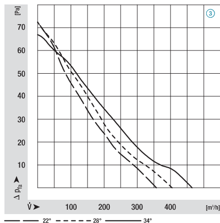
M4Q045-CA01-**, Ø 200, 50 Hz
