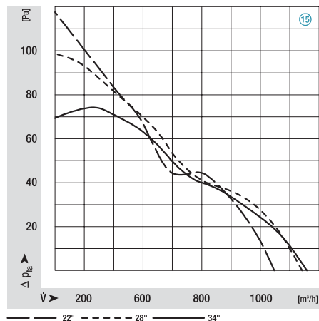
M4Q045-EF01-**-**, Ø 300, 50 Hz
