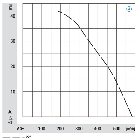
M4Q045-CA01-**, Ø 230, 60 Hz
