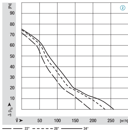
M4Q045-BD01-**, Ø 154, 60 Hz
