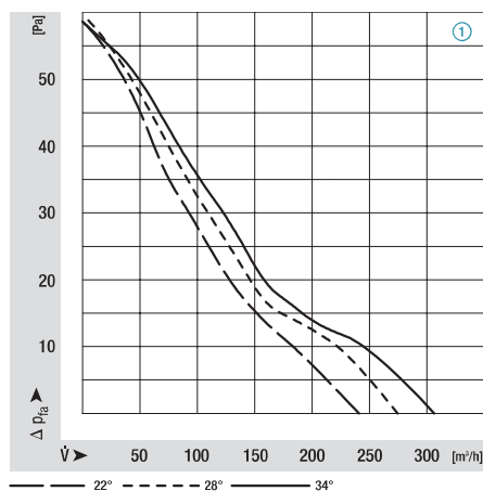
M4Q045-BD01-**, Ø 172, 50 Hz
