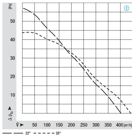
M4Q045-BD01-**, Ø 200, 60 Hz
