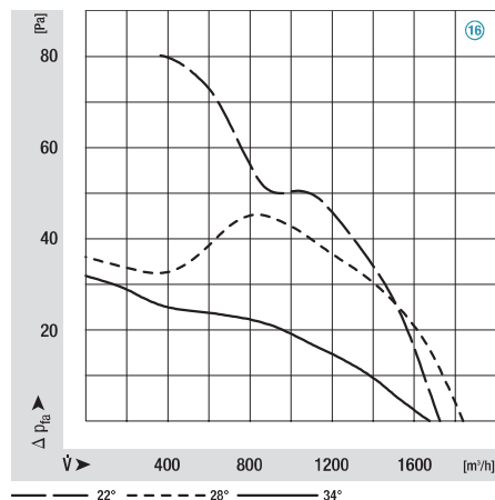
M4Q045-EF01-**-**, Ø 300, 60 Hz
