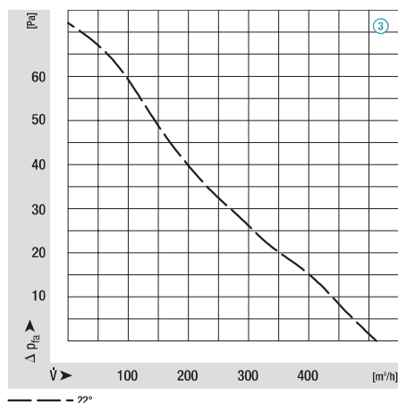
M4Q045-CA01-**, Ø 230, 50 Hz
