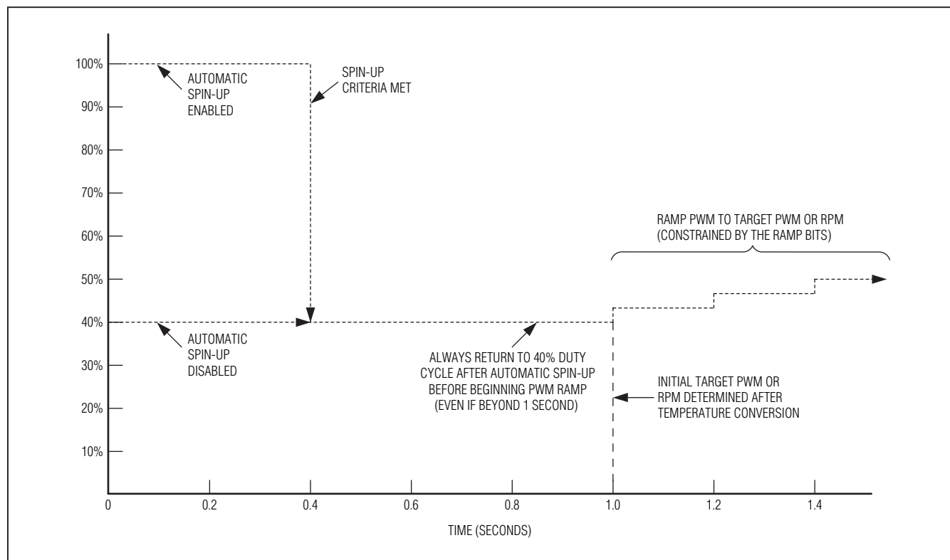
Figure 3. Fan Spin-Up
