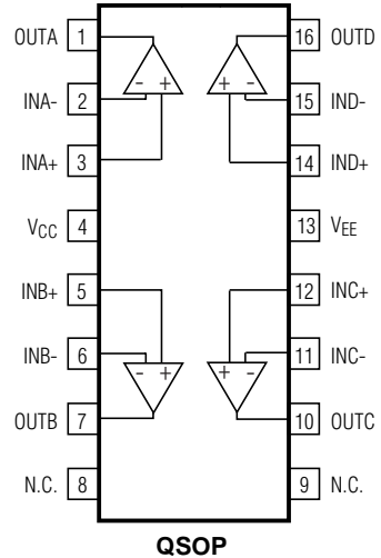
MAXIM MAX4284
