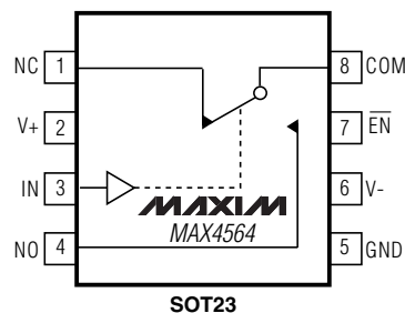
SOT23
