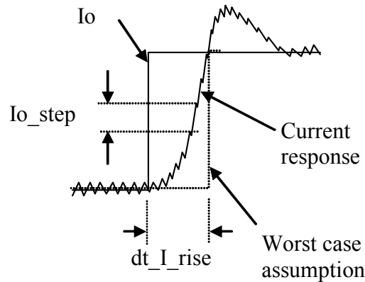
Figure 8. Transient Parameters
