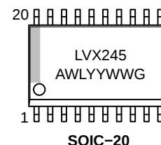
SOIC-20
