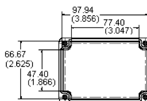
Lid - Inside
