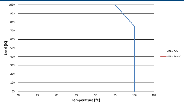
MGJ1D241505MPC
