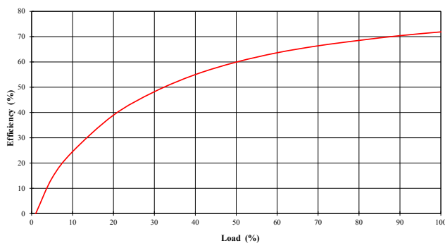
MGJ1D121905MPC
