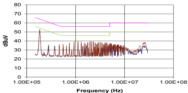
MGJ1D241509MPC
