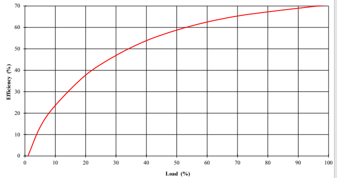
MGJ1D241505MPC
