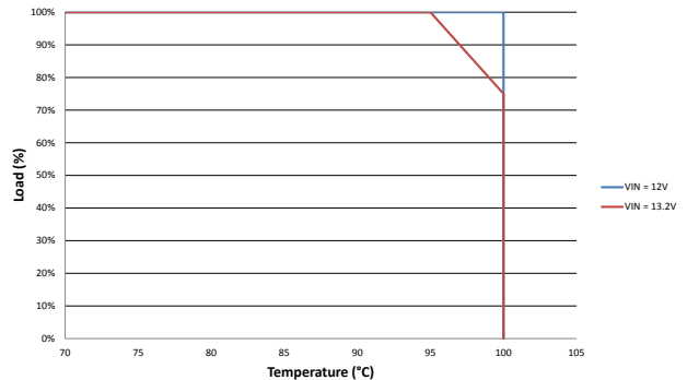
MGJ1D121905MPC
