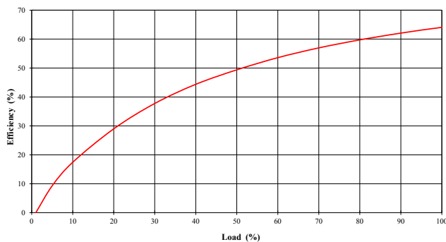
MGJ1D121505MPC
