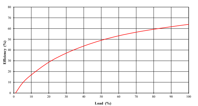
MGJ1D241509MPC
