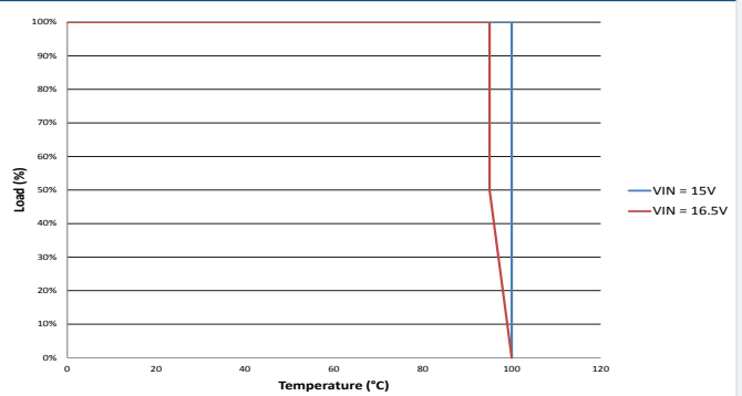
MGJ1D151509MPC
