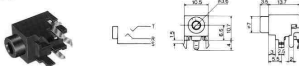
No.MX-362GL (φ3.5) STEREO
