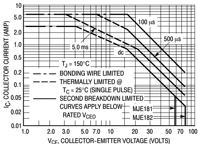
Figure 6. MJE181, MJE182
