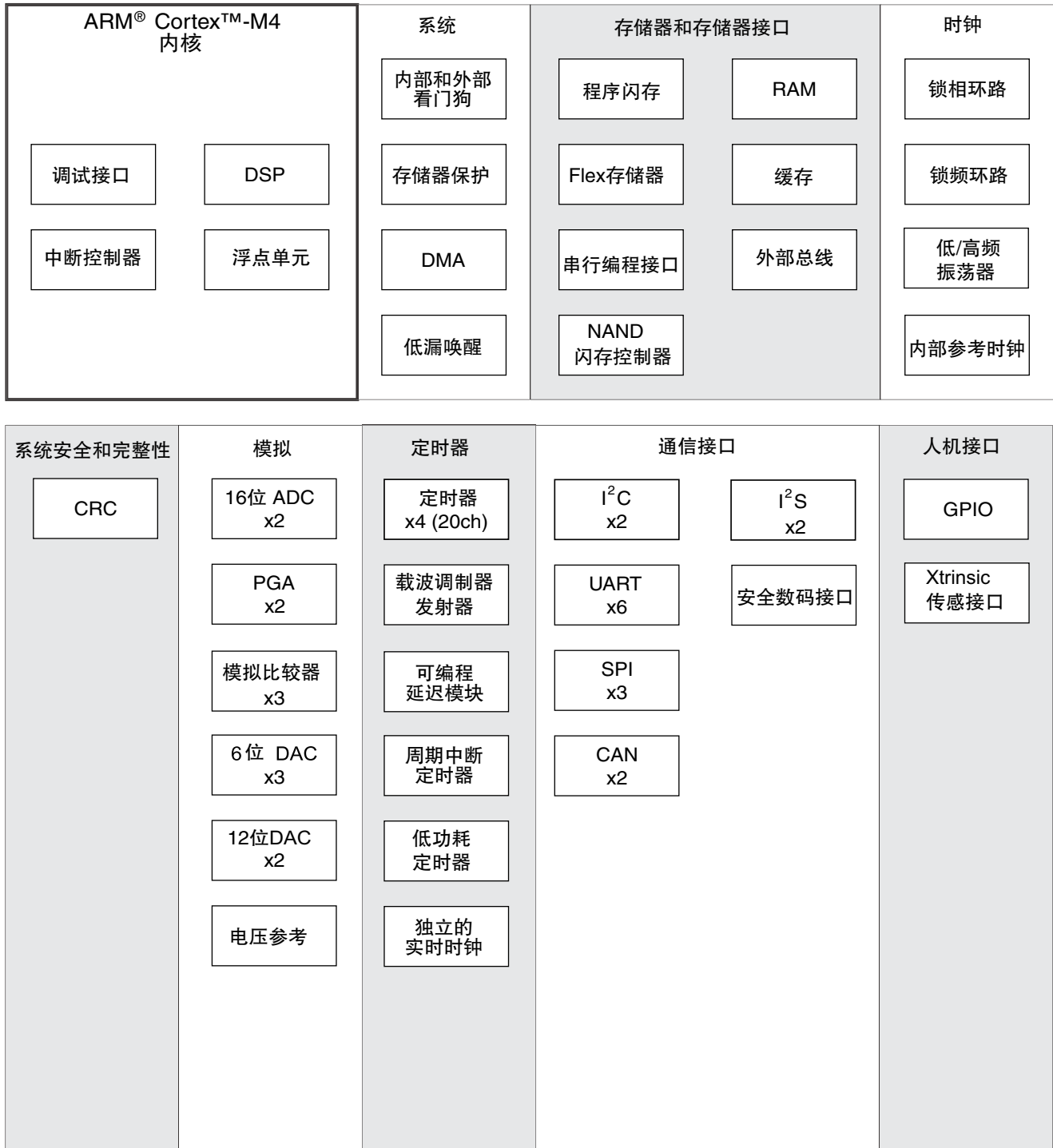
图 3. K10 模块结构图
