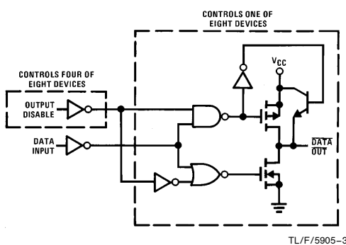
MM54C244/MM74C244
