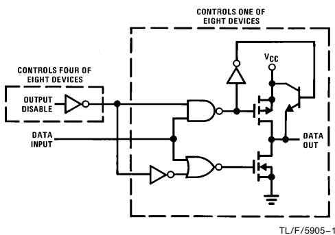
MM54C240/MM74C240
