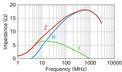
MMZ1608R121ATD25
