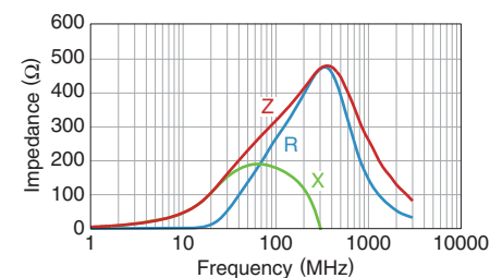
MMZ1608Y301BTD25
