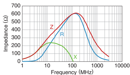
MMZ1608R601ATD25
