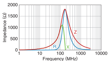
MMZ1608Q102BTD25
