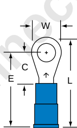
MNG14-10R/L Stud Size 10 Wire Range 16-14
