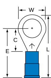
MNG14-516R/S Stud Size 5/16 Wire Range 16-14
