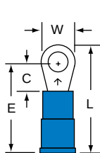
MNG14-6R/S Stud Size 6 Wire Range 16-14
