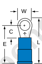
MNG14-8R/S Stud Size 8 Wire Range 16-14
