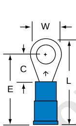
MNG14-10R Stud Size 10 Wire Range 16-14
