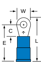
MNG14-4R/S Stud Size 4 Wire Range 16-14
