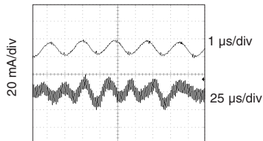
MOR2812D Input Ripple (lin)
