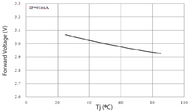
T j --Forward Voltage
