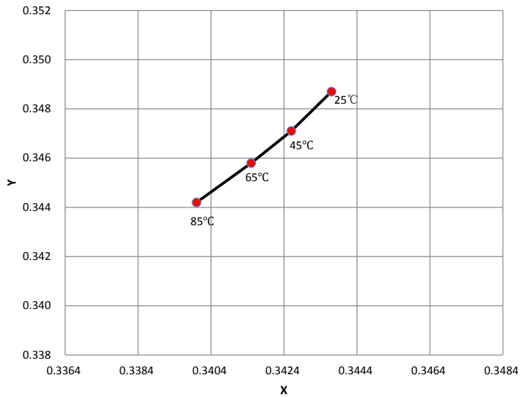
T_s vs. CIE x, y Shift
