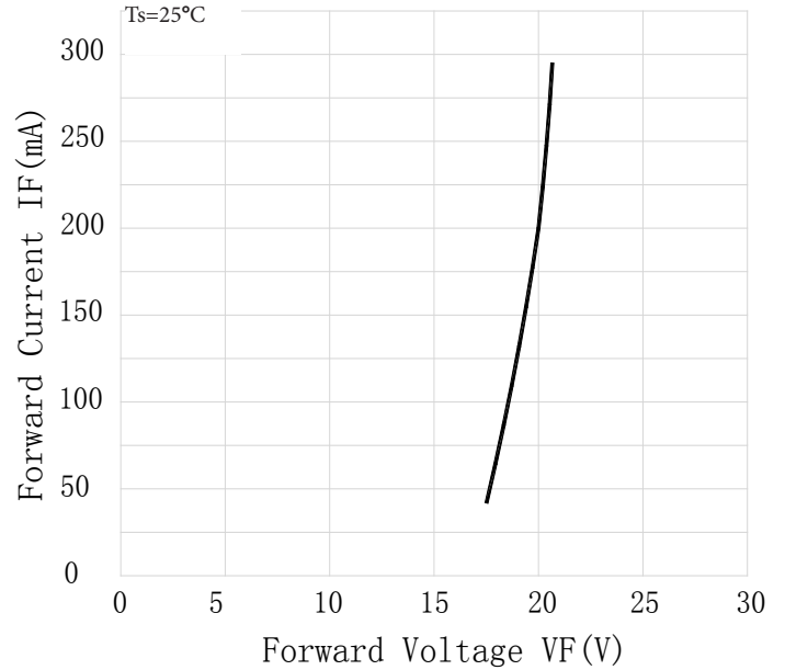
V_f ----- I_f
