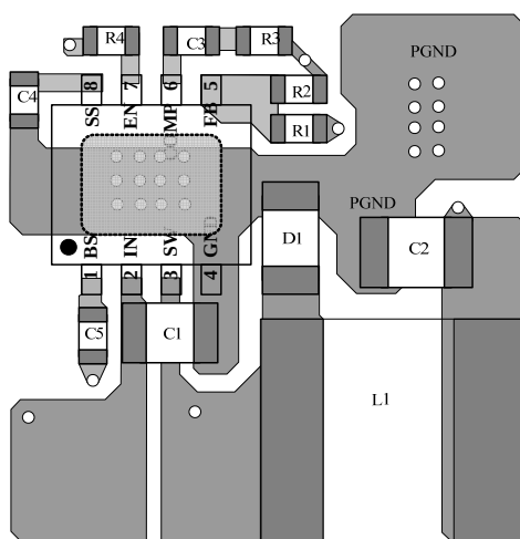
Top Layer
