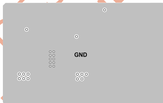
Inner Layer2
