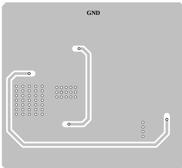
Bottom Layer
