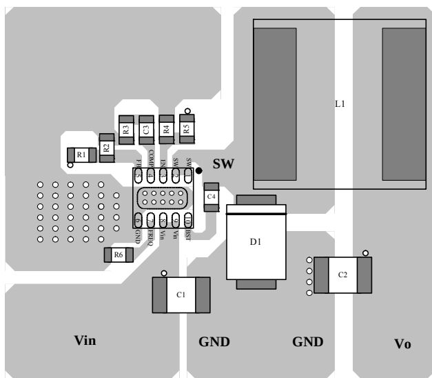
TOP Layer
