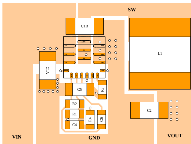
Top Layer
