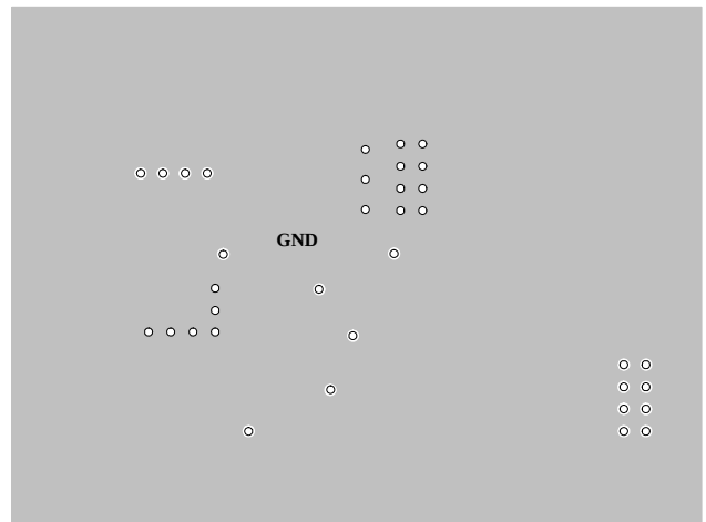
Inner2 Layer
