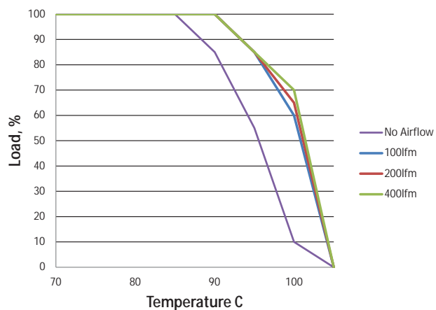
MTC2S1203MC - 18Vin
