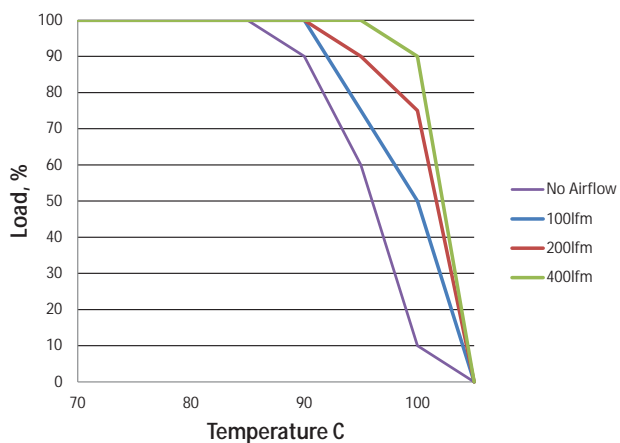
MTC2S1203MC - 9Vin
