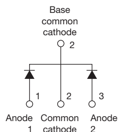
VS-MURB1620CTPbF
